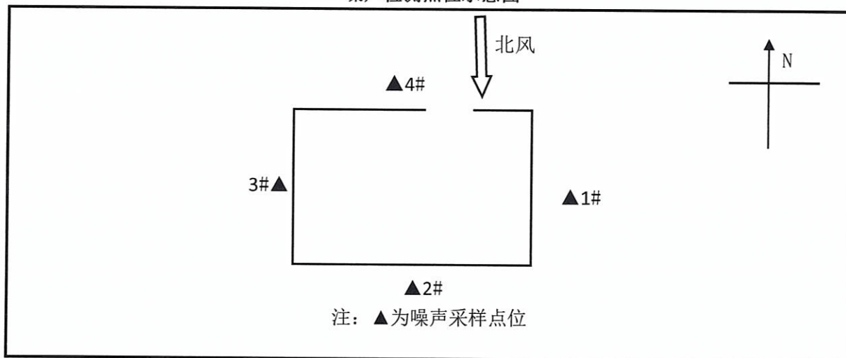
噪声检测点位示意图
